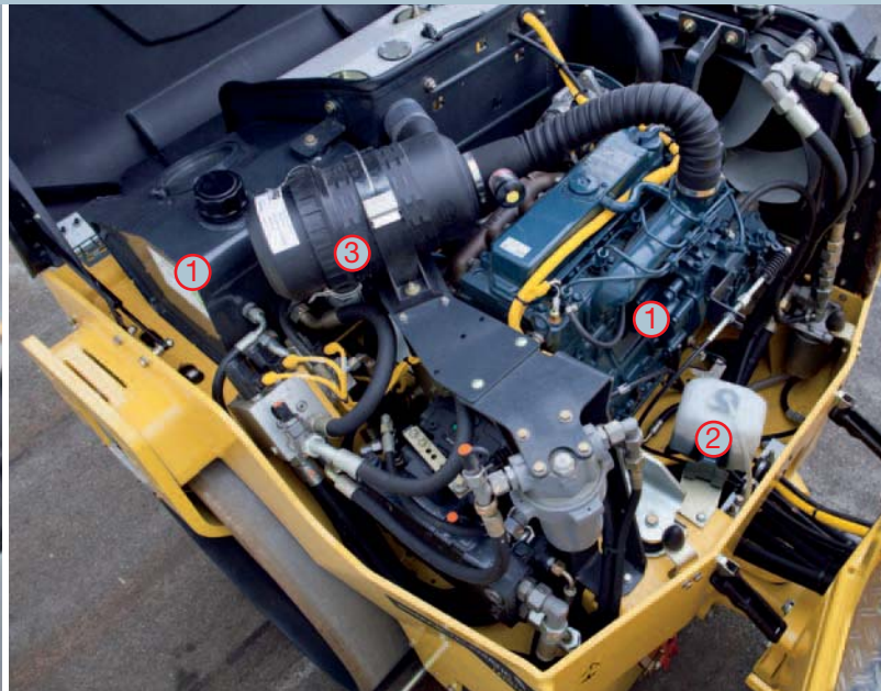
Easy-Check-Konzept: Öl (1), Wasser (2), Luft (3) – einfach erreichbar, schnell startklar.
